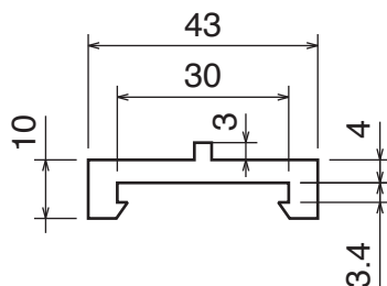
Profilo ad "U" / U-profile / U-Profil
